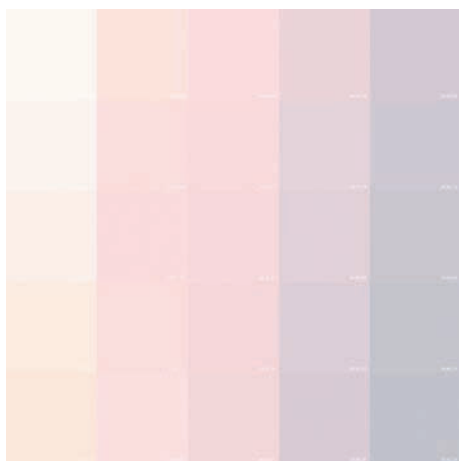
sommer licht weiss 2020/34 – 2020 30.6.2013 – 20:35:27 – 20:42:31
